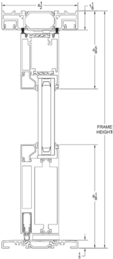
Pivot Door Cross Section
